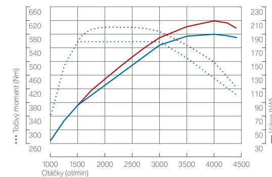
Hodnoty výkonu modelu BMW 330d s BMW M Performance Power Kit Plné zatížení 330d
